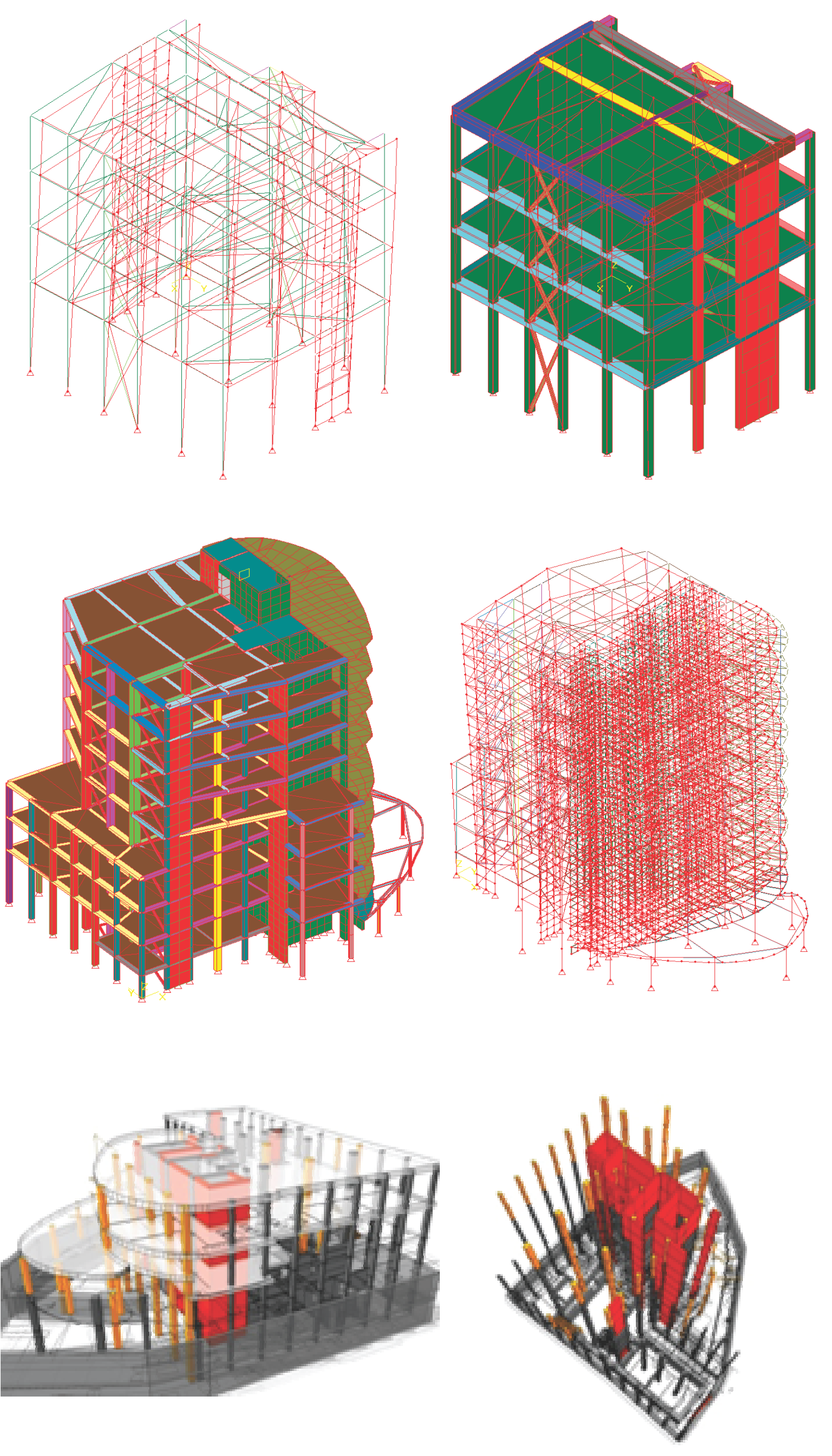
immagini di modello esportabile con protocollo IFC
