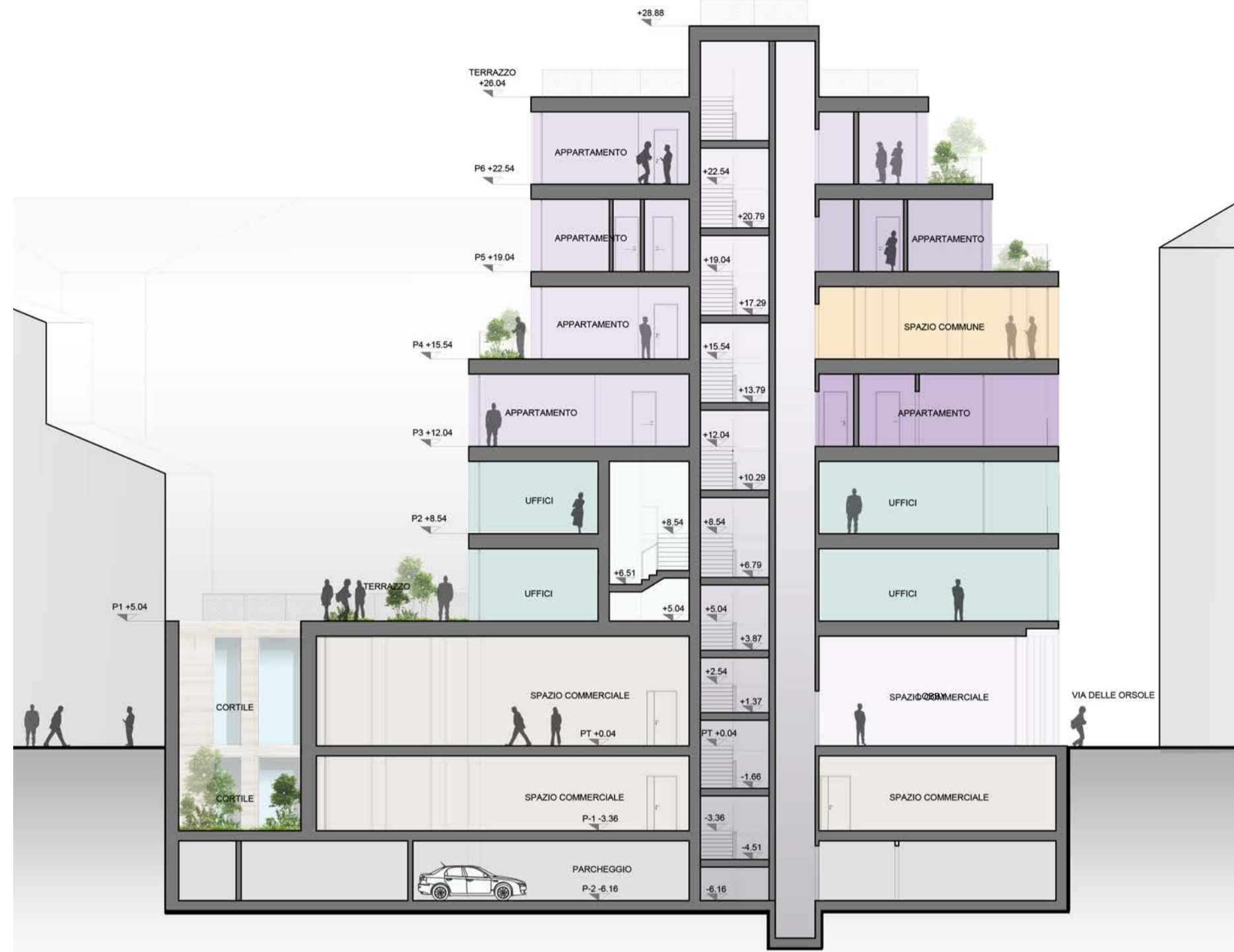
Sezione B-B 1:200
