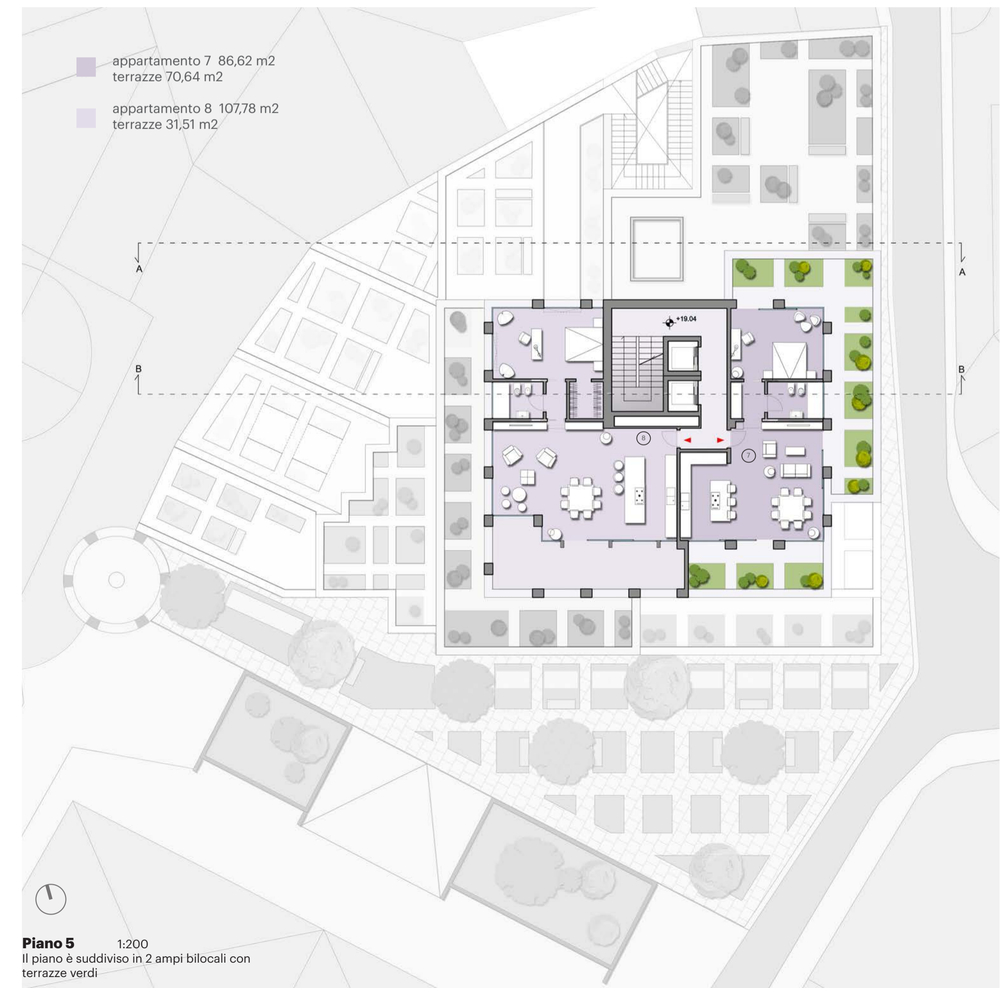
Piano 3 1:200 Il piano è suddiviso in 4 appartamenti, bilocali e trilocali con ampie terrazze verdi
